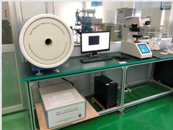
纯铁矫顽力测试仪
